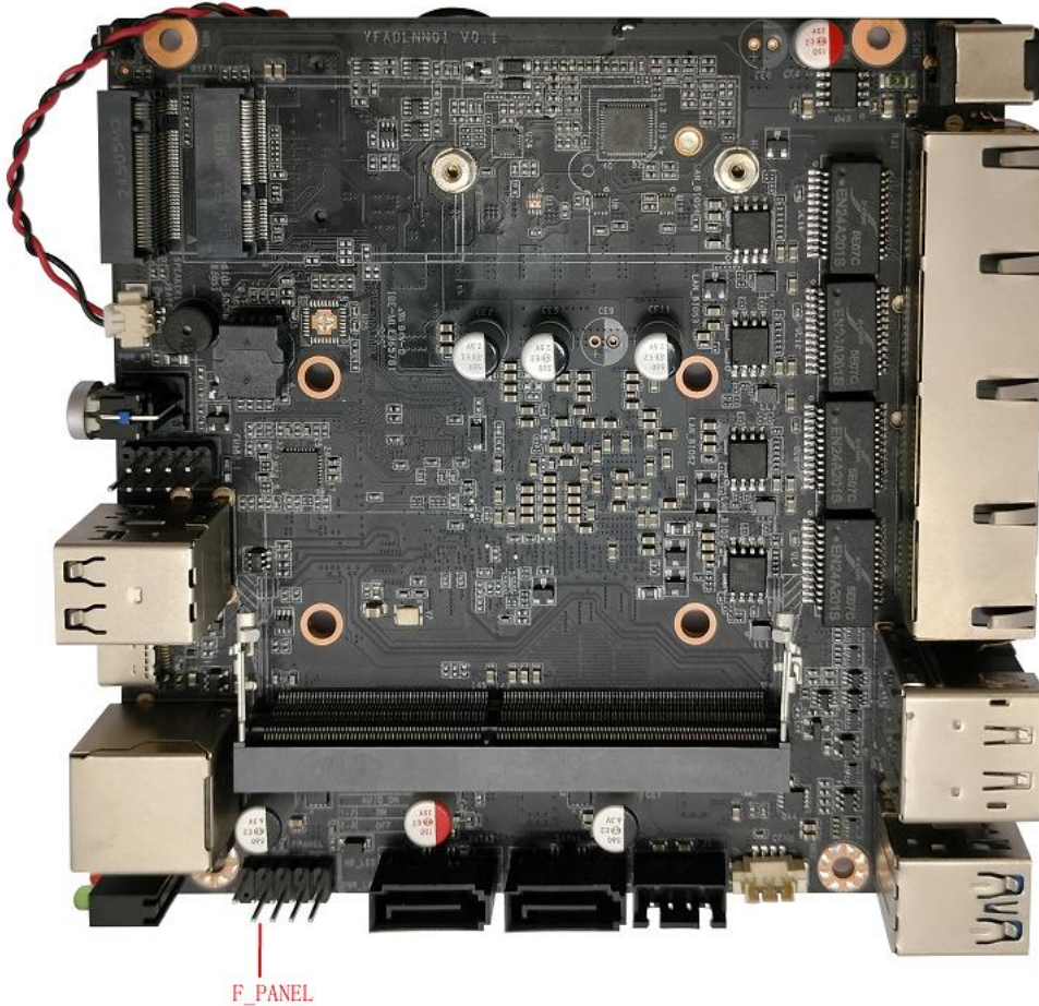
F_PANEL (2×5 pin 间距 2.54mm 第 10 pin 空)
