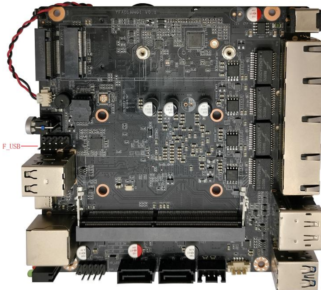
F_USB1 (2×5 pin 间距 2.54mm 第 9 pin 空)
